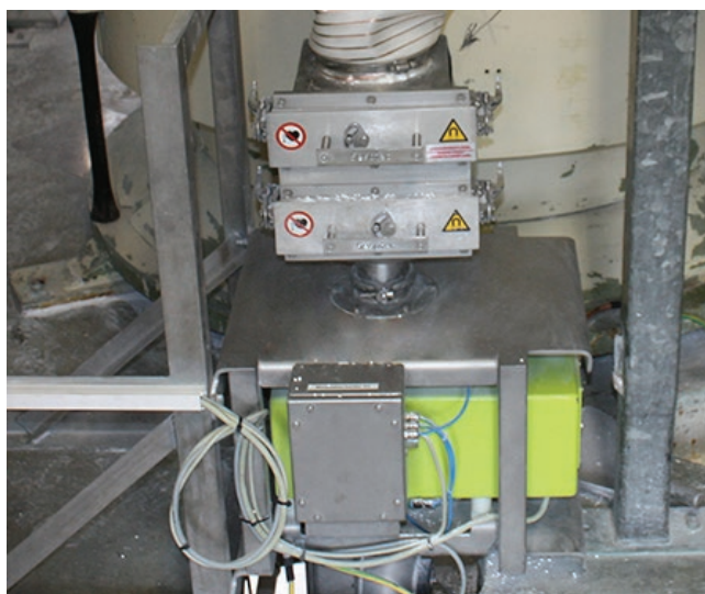
» Magnetski separator MAGBOX ispred induktivnog separatora metala RAPID PRO-SENSE (komponenta zelene boje) zadržava željezne čestice i tako rasterećuje induktivnu separaciju. | Izvor: Sesotec
